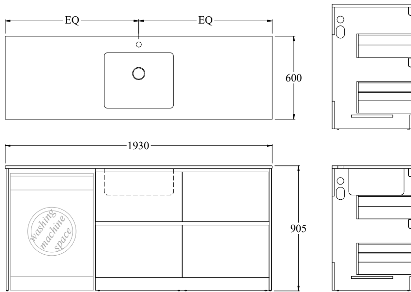
LEV19RDRDRCCCEL | LEV19RDRDRCCMW
